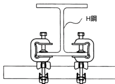
足場自在金物 水平用 M-2型
