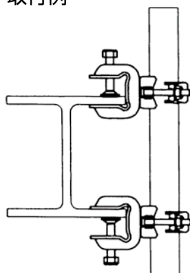
足場自在金物 垂直用 M-1型
