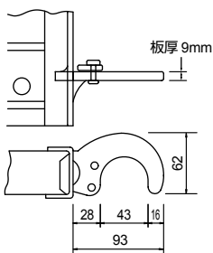
フック部寸法 (mm)
