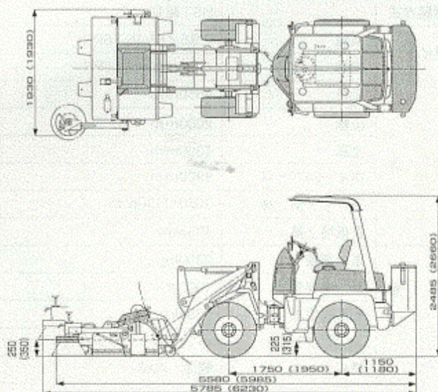
■全体図 (単位:mm)
