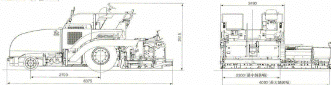
■全体図 (単位:mm)
