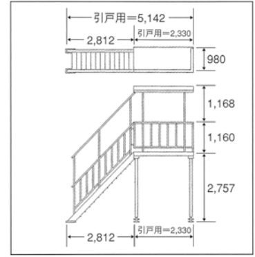
アルミ階段寸法図
